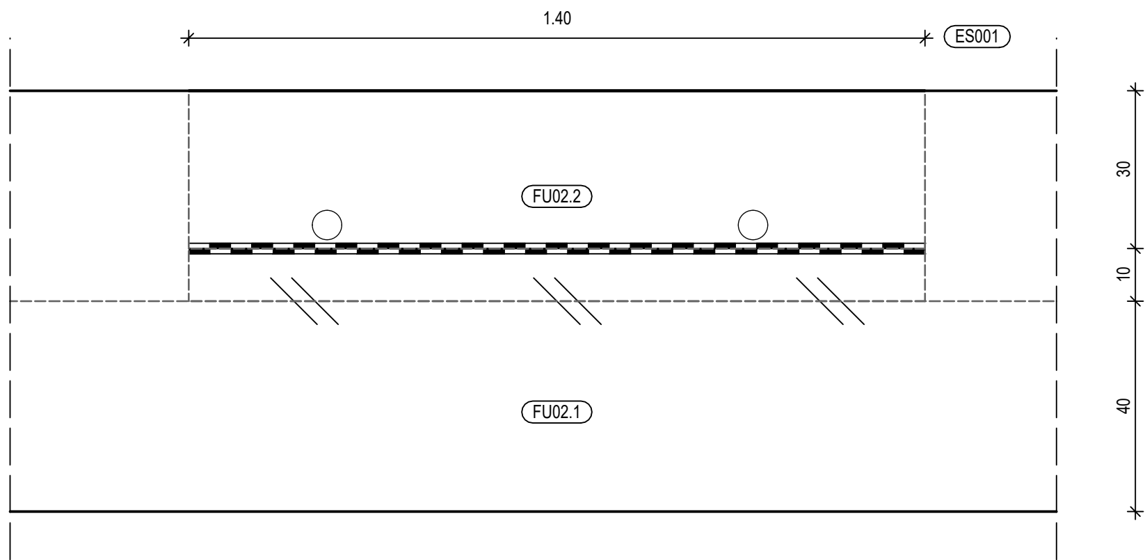
Detail 1 Großflächengleitfolie M1:10 Oberfläche Aufkantung FU02.1 Flügelgeglättet!
